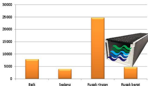
Gambar 4. Saluran Irigasi Primer Tahun 2022
