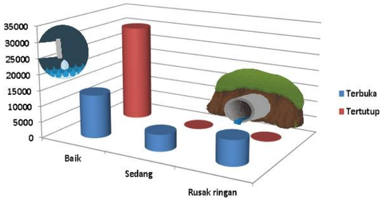
Gambar 5. Kondisi Drainase Kota Lubuklinggau Tahun 2022
