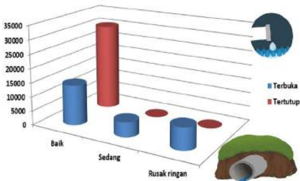
Gambar 5. Kondisi Drainase Kota Lubuklinggau Tahun 2023
